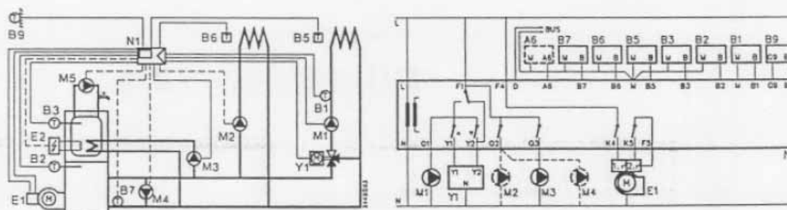
Obr. 5.11 2-stupňový hořák, směšovací topný okruh, TUV a jeden další výstup (čerpadlový topný okruh, cirkulační čerpadlo TUV, el. topná vložka, čerpadlo ochozu kotle)
