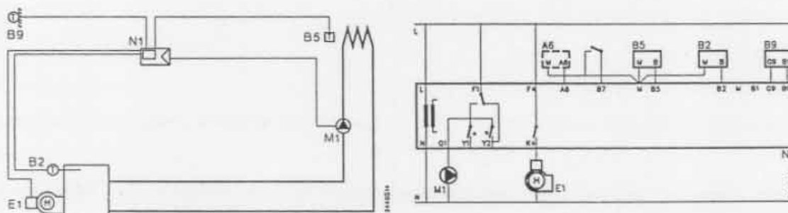
Obr. 5.2 1-stupňový hořák a čerpadlový topný okruh
