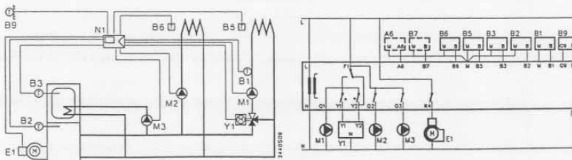
Obr. 5.6 1-stupňový hořák, směšovací topný okruh, čerpadlový topný okruh a TUV
