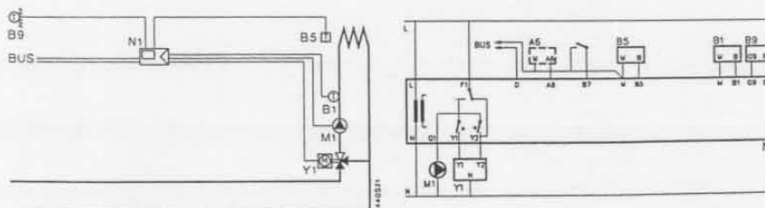
Obr. 5.3 Směšovací topný okruh
